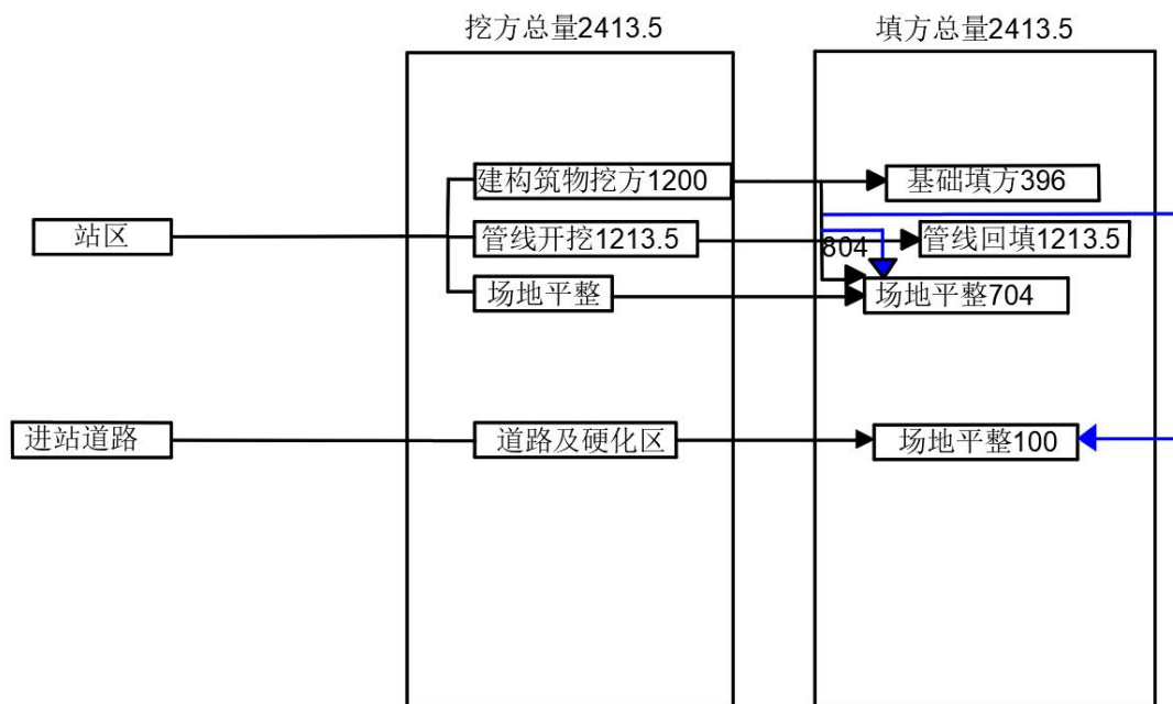
图 1-2 工程土石方流向框图 单位: \text{m}^3
